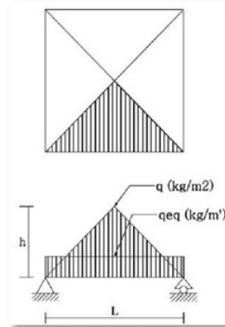
Gambar 4. Perubahan Beban Segi Tiga Ke Beban Garis
