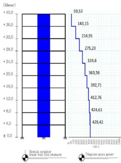
(c) Gambar 6. Diagram Gaya Geser Terhadap Ketinggian Gedung (A) Model 1 (B) Model 2 dan (C) Model 3
