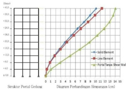
Gambar 7. Diagram Perbandingan Simpangan (Model 1, 2, dan 3)
