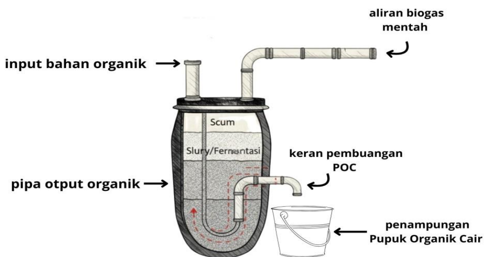
Gambar Eco Power untuk produksi biogas dan POC
