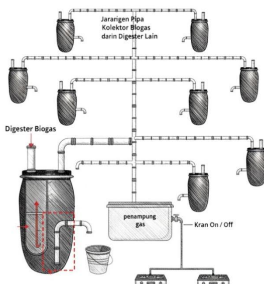
Gambar Cara kerja Eco Power
