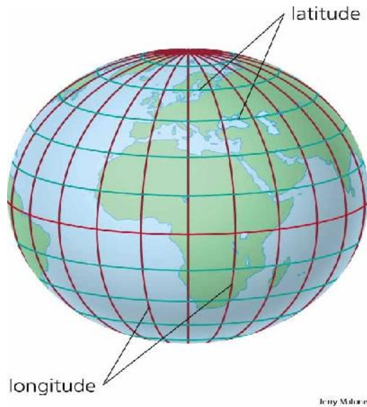
Gambar 1. Lintang (Latitude) dan bujur (Longitude)
